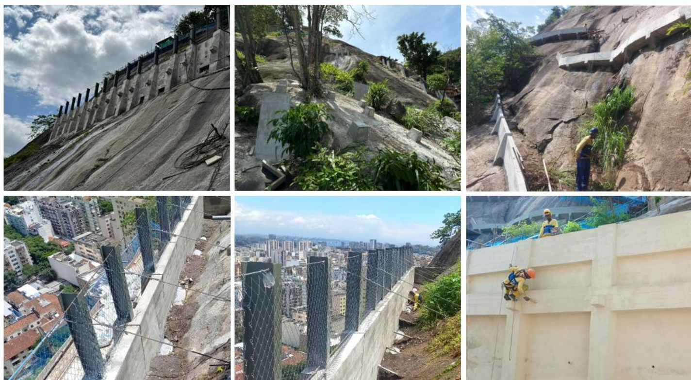
OBRAS EMERGENCIAIS DE CONTENÇÃO DE ENCOSTA ENCOSTA RUA OSCAR PIMENTEL TIJUCA
