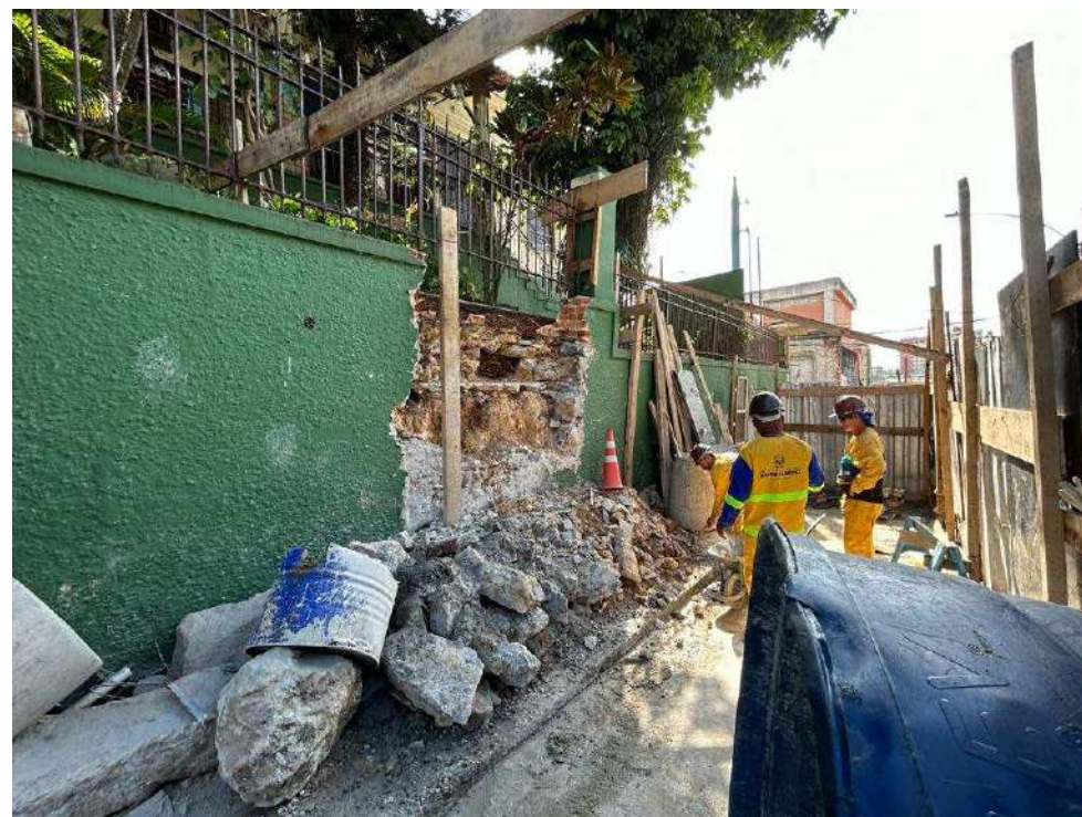
Execução da cortina ancorada e ao lado demolição parcial de muro existente
