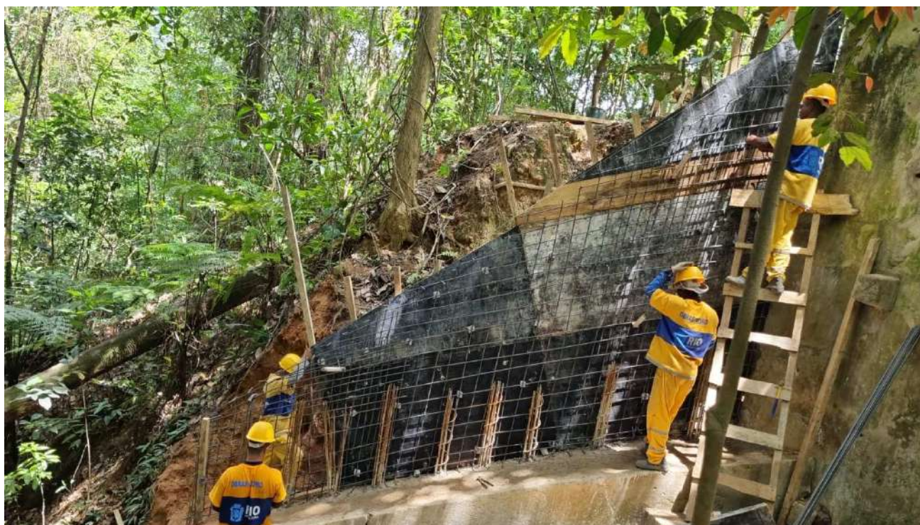
Execução de cortina ancorada
